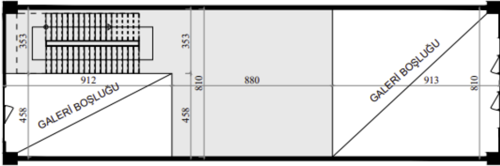
1.NORMAL KAT
