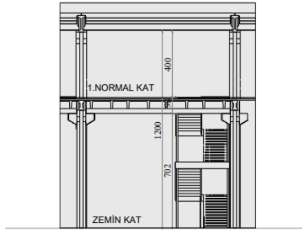
ŞEMATİK KESİT
