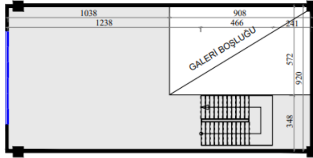
1.NORMAL KAT
