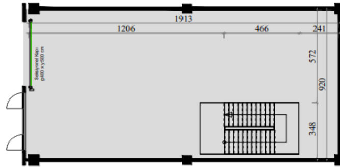
ZEMİN KAT
