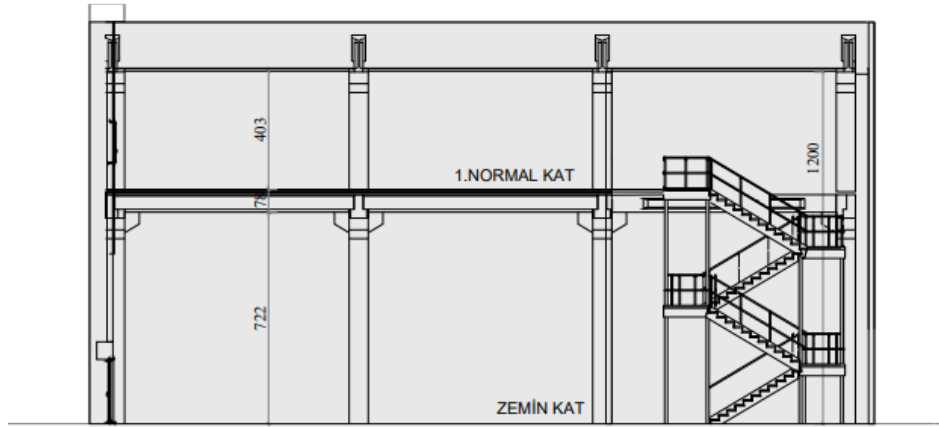
ŞEMATİK KESİT
