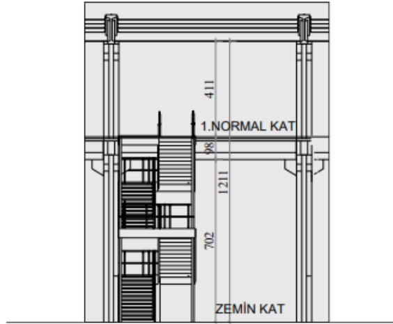
ŞEMATİK KESİT
