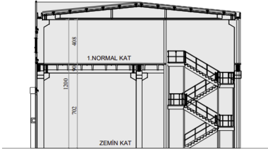
ŞEMATİK KESİT
