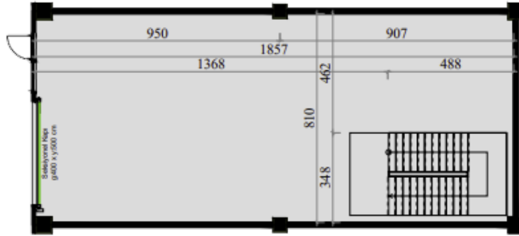
ZEMİN KAT
