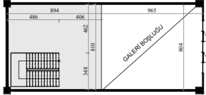
1.NORMAL KAT
