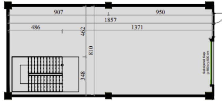
ZEMİN KAT
