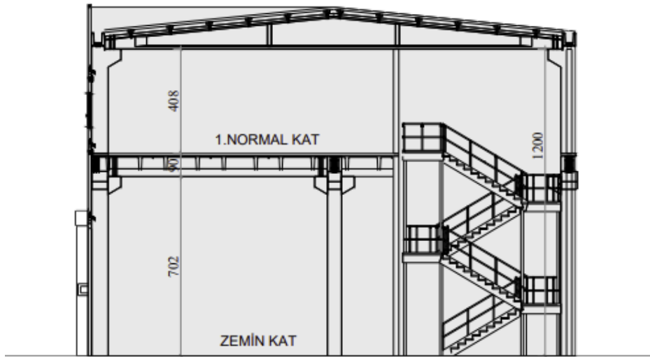
ŞEMATİK KESİT
