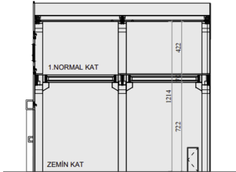
ŞEMATİK KESİT
