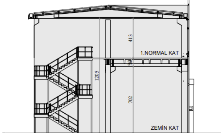
ŞEMATİK KESİT
