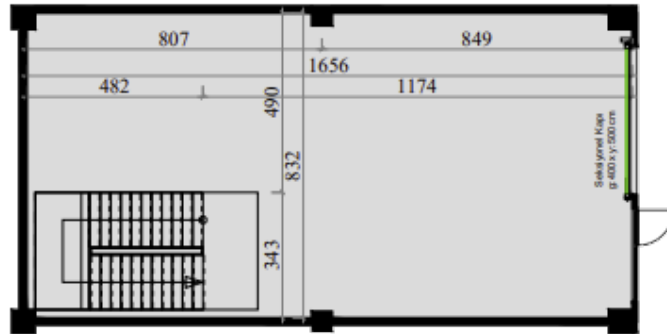
ZEMİN KAT
