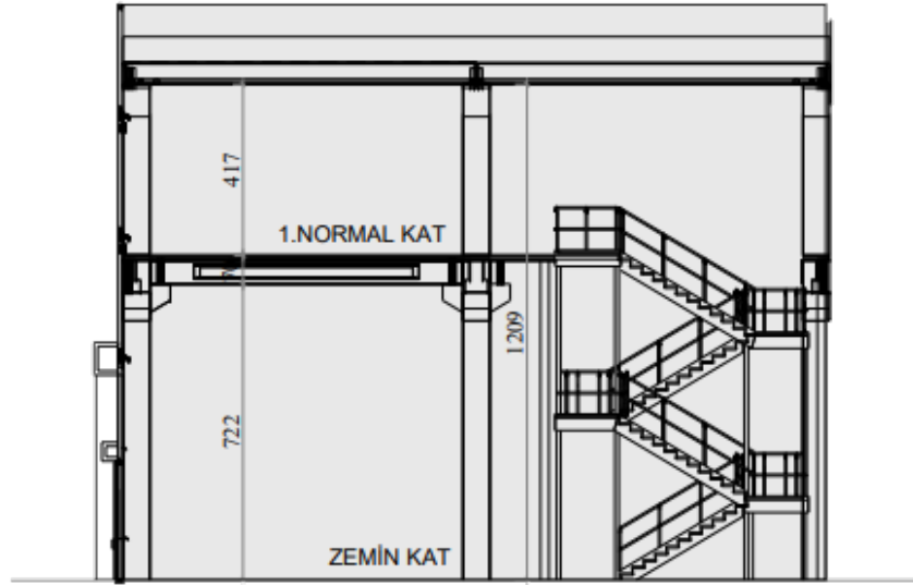
ŞEMATİK KESİT
