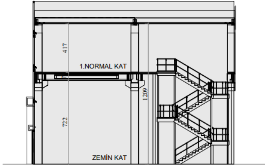
ŞEMATİK KESİT
