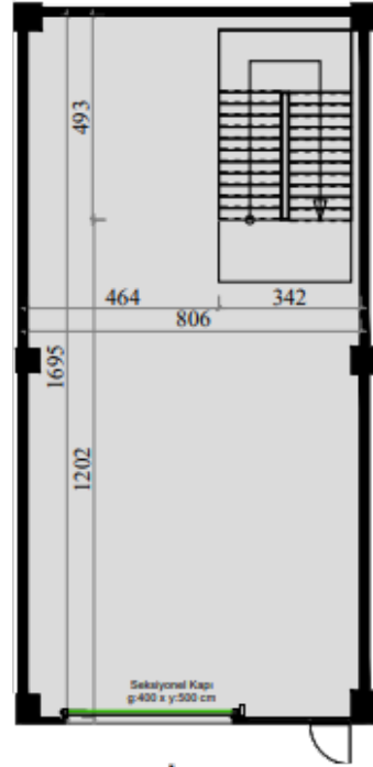
ZEMİN KAT
