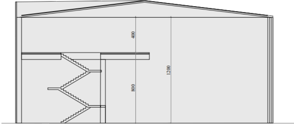
ŞEMATİK KESİT
