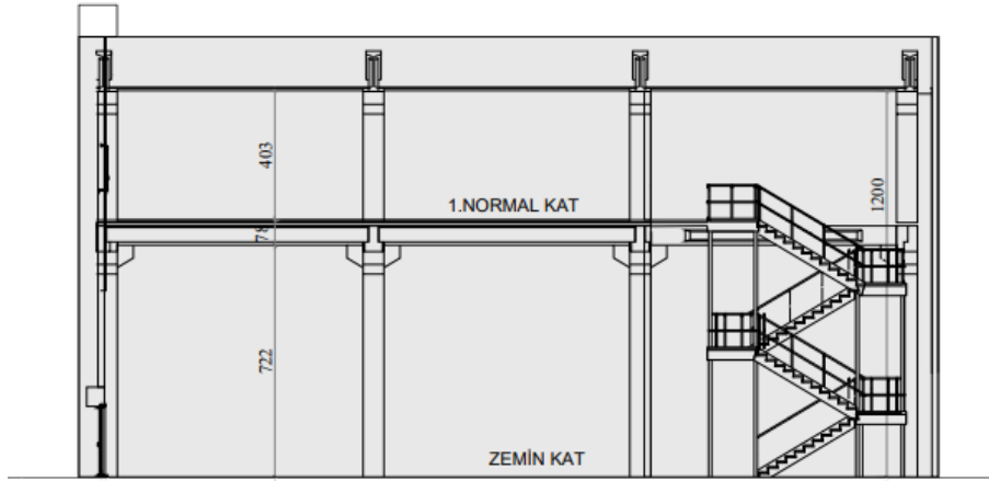
ŞEMATİK KESİT
