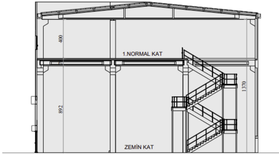
ŞEMATİK KESİT
