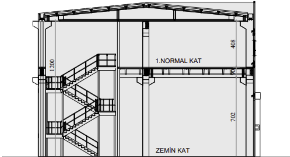
ŞEMATİK KESİT
