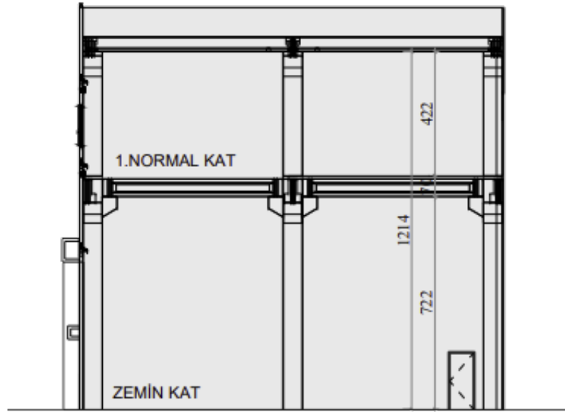
ŞEMATİK KESİT
