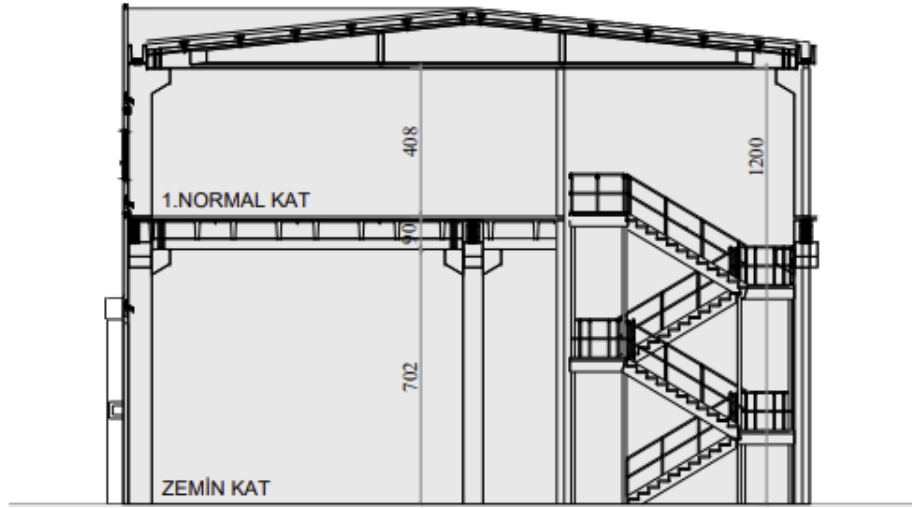
ŞEMATİK KESİT
