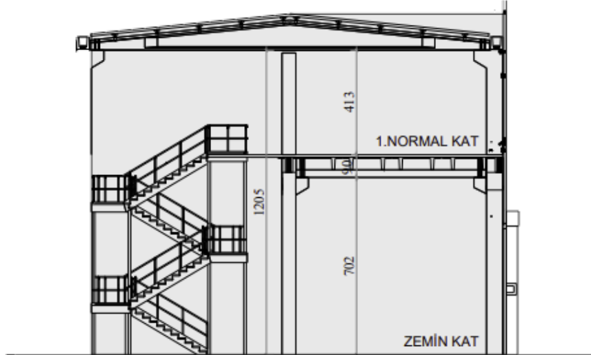
ŞEMATİK KESİT
