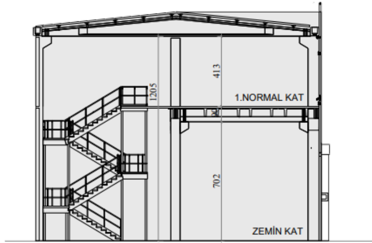
ŞEMATİK KESİT
