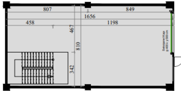
ZEMİN KAT
