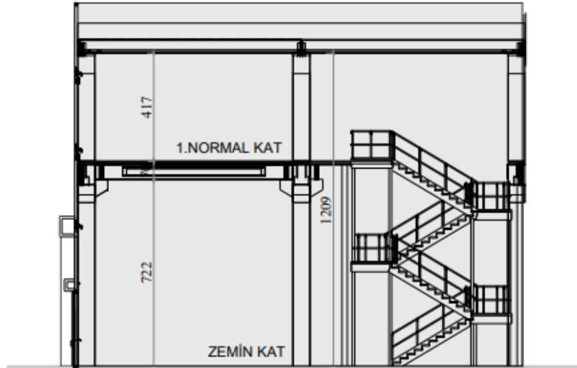
ŞEMATİK KESİT
