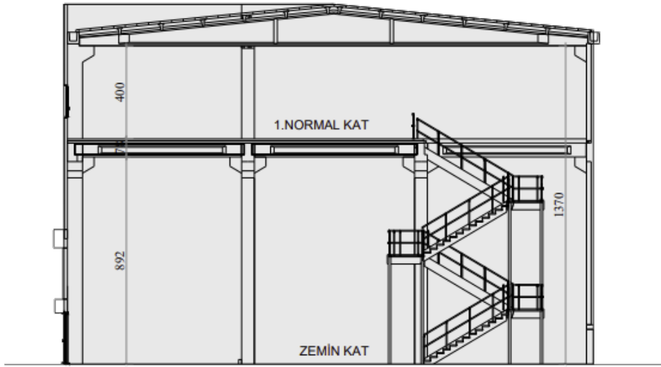
ŞEMATİK KESİT
