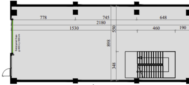
ZEMİN KAT
