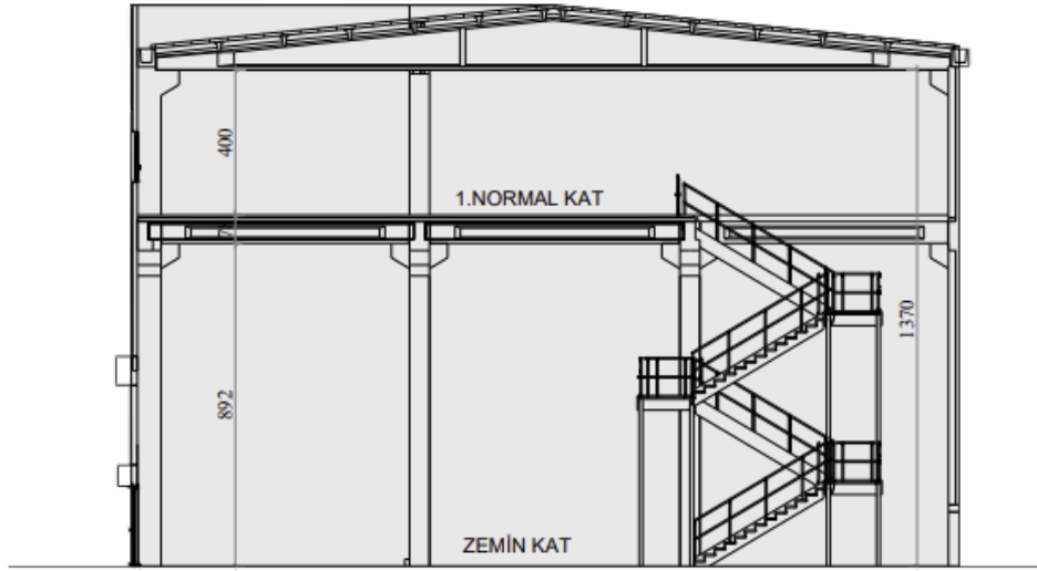
ŞEMATİK KESİT
