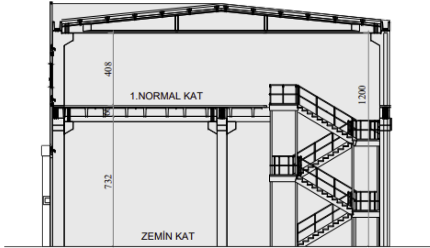
ŞEMATİK KESİT
