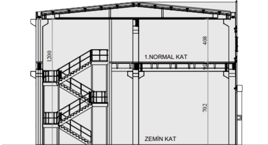
ŞEMATİK KESİT
