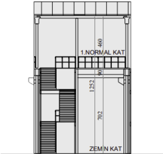
ŞEMATİK KESİT
