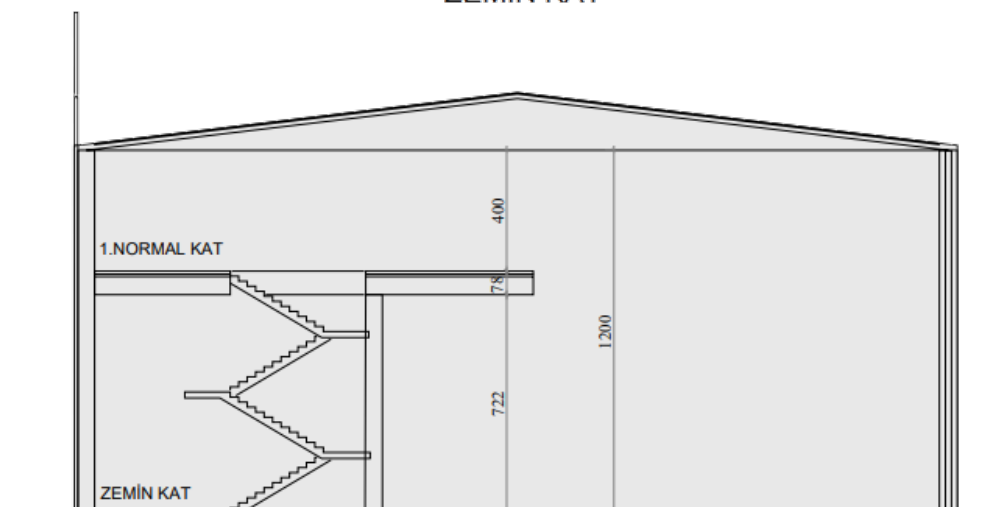
ŞEMATİK KESİT
