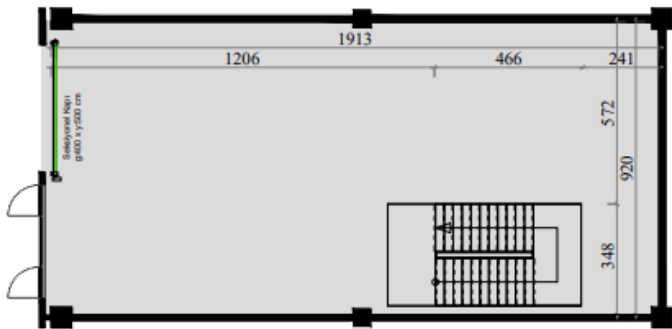
ZEMİN KAT
