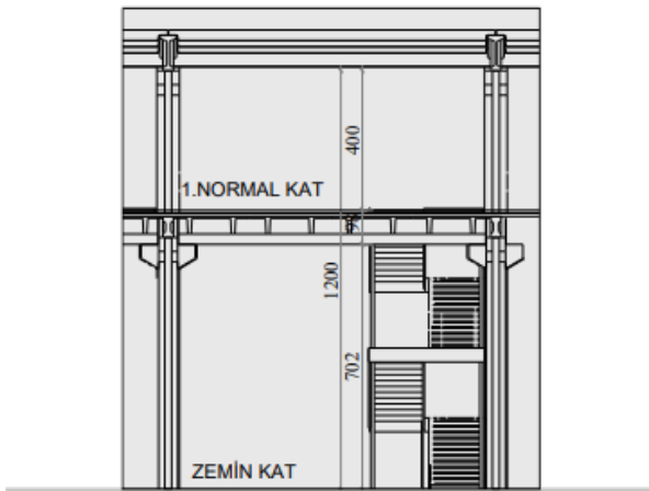
ŞEMATİK KESİT
