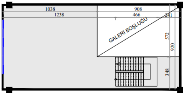
1.NORMAL KAT
