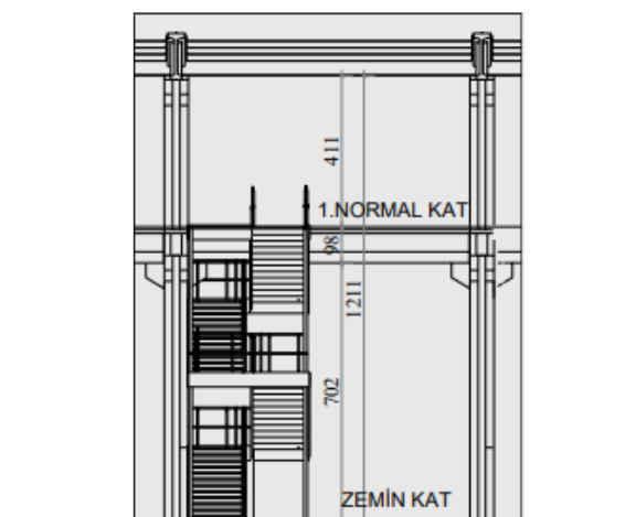
ŞEMATİK KESİT
