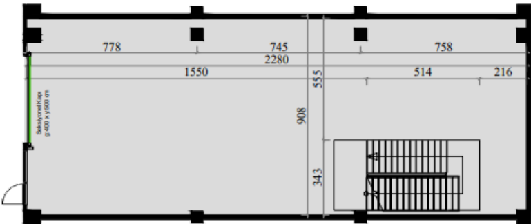
ZEMİN KAT
