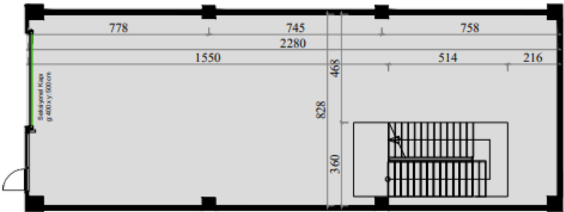
ZEMİN KAT
