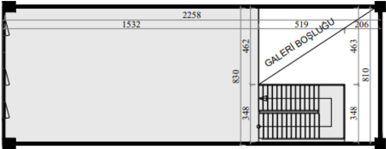
1.NORMAL KAT
