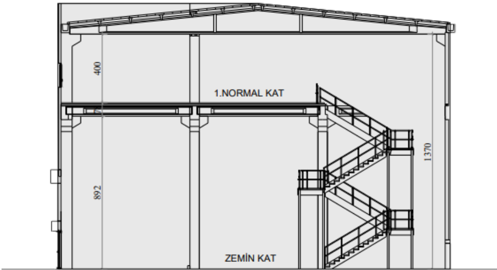
ŞEMATİK KESİT
