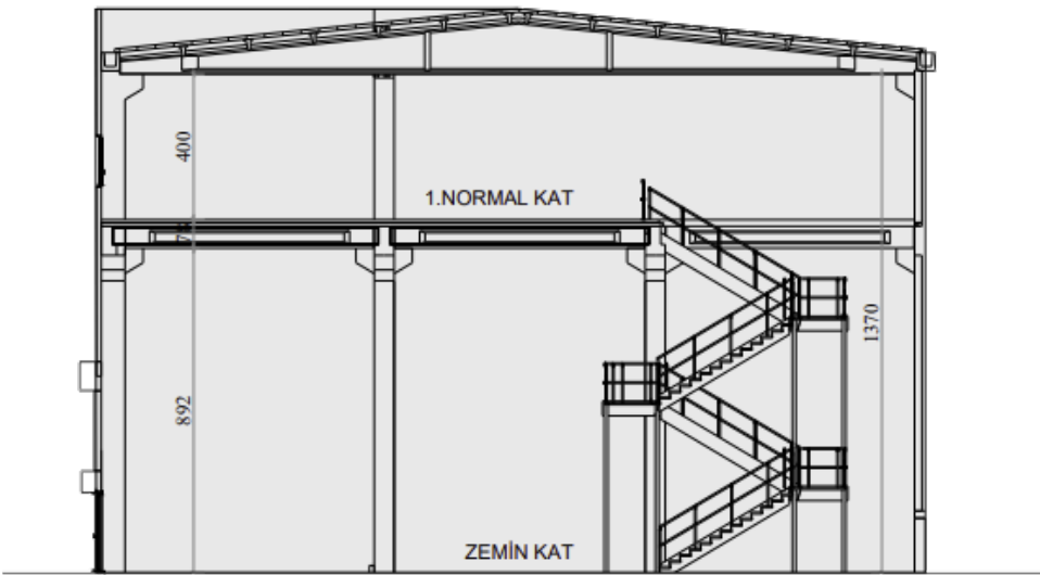
ŞEMATİK KESİT
