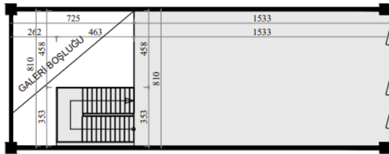
1.NORMAL KAT
