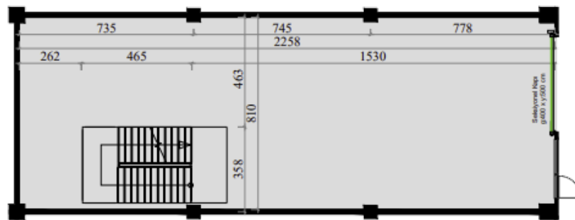
ZEMİN KAT
