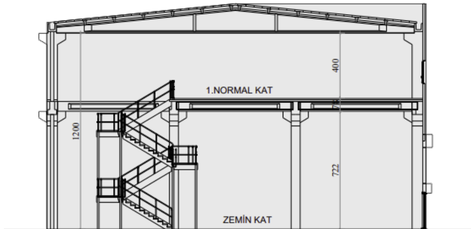
ŞEMATİK KESİT
