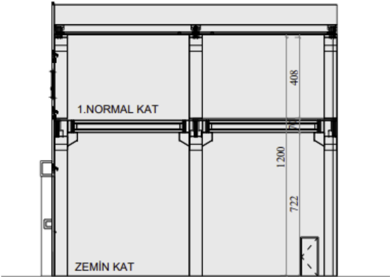
ŞEMATİK KESİT
