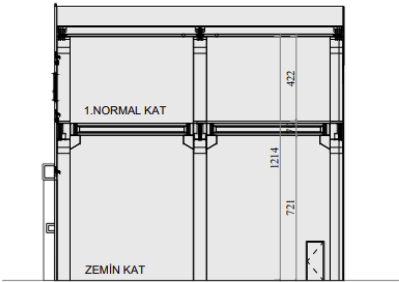
ŞEMATİK KESİT
