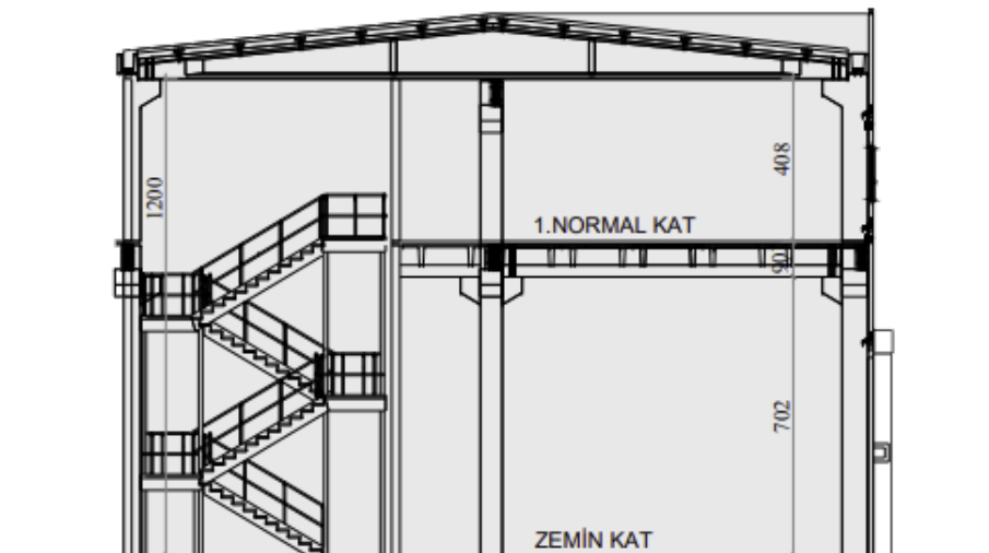
ŞEMATİK KESİT
