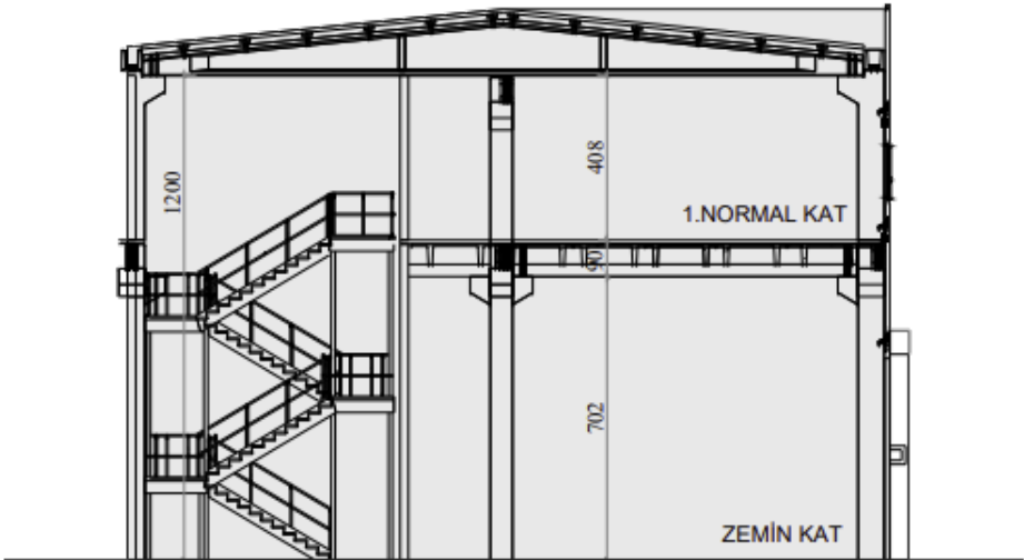
ŞEMATİK KESİT
