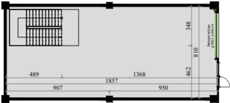
ZEMİN KAT
