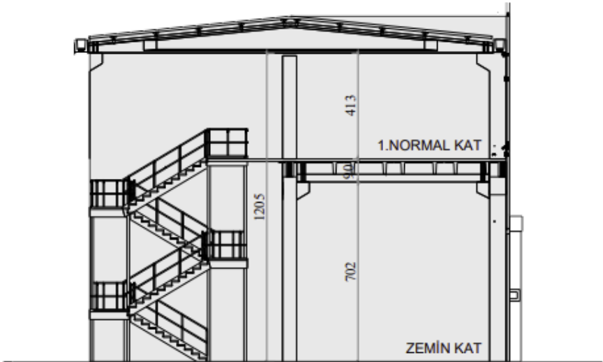
ŞEMATİK KESİT
