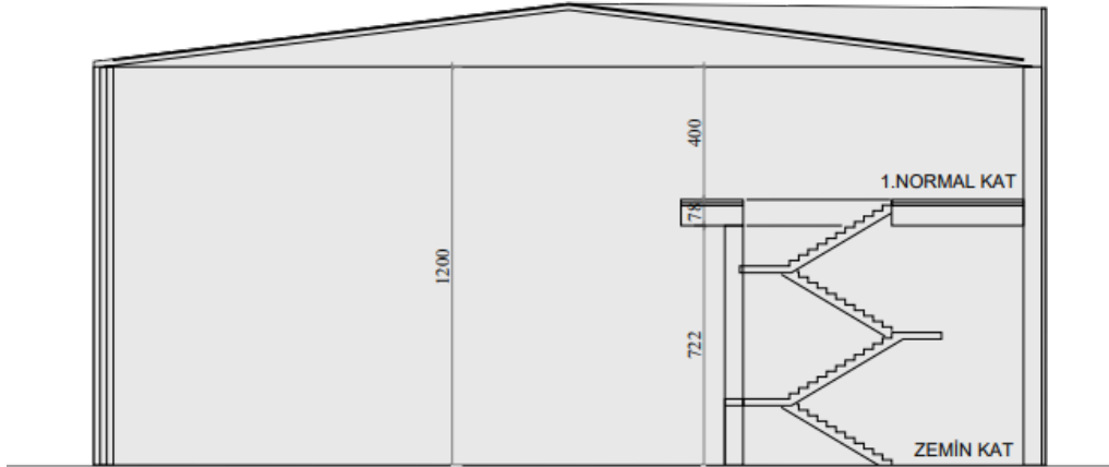
ŞEMATİK KESİT
