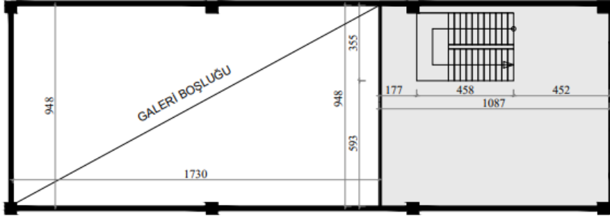
1.NORMAL KAT
