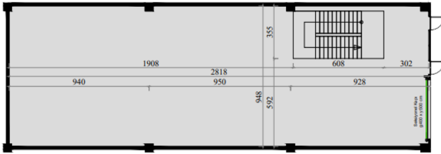
ZEMİN KAT
