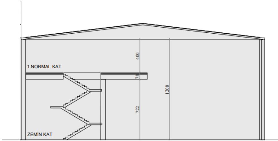
ŞEMATİK KESİT
