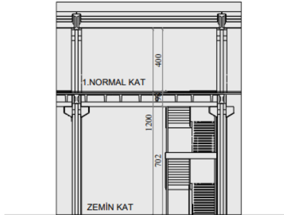
ŞEMATİK KESİT
