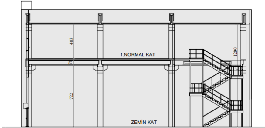
ŞEMATİK KESİT
