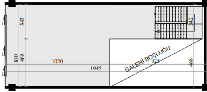
1.NORMAL KAT
