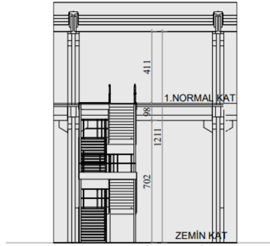
ŞEMATİK KESİT
