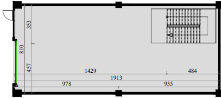
ZEMİN KAT
