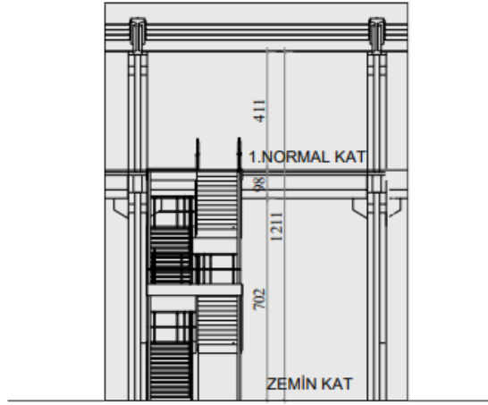
ŞEMATİK KESİT
