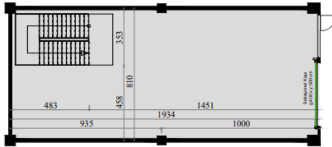
ZEMİN KAT
