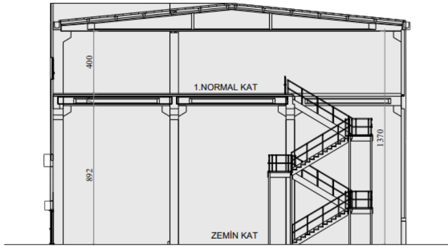
ŞEMATİK KESİT
