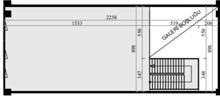
1.NORMAL KAT
