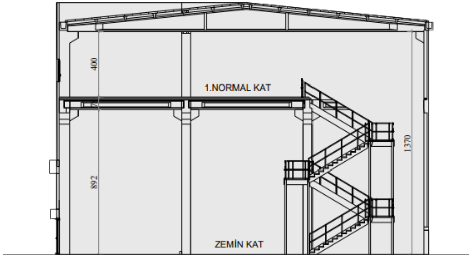
ŞEMATİK KESİT
