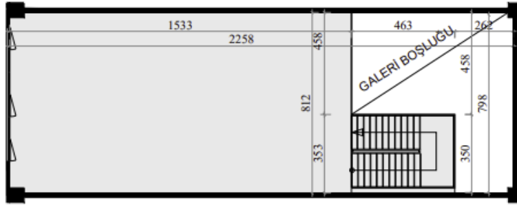
1.NORMAL KAT
