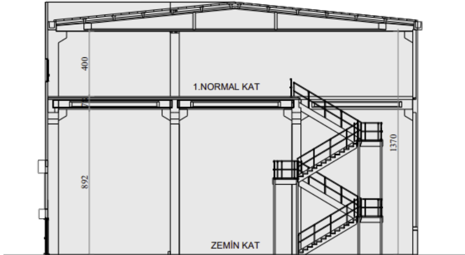
ŞEMATİK KESİT
