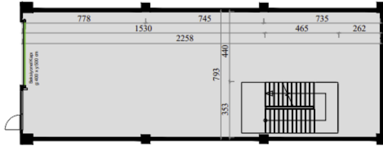
ZEMİN KAT
