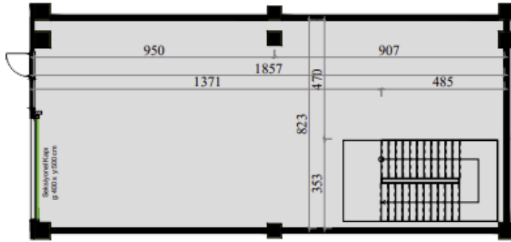
ZEMİN KAT
