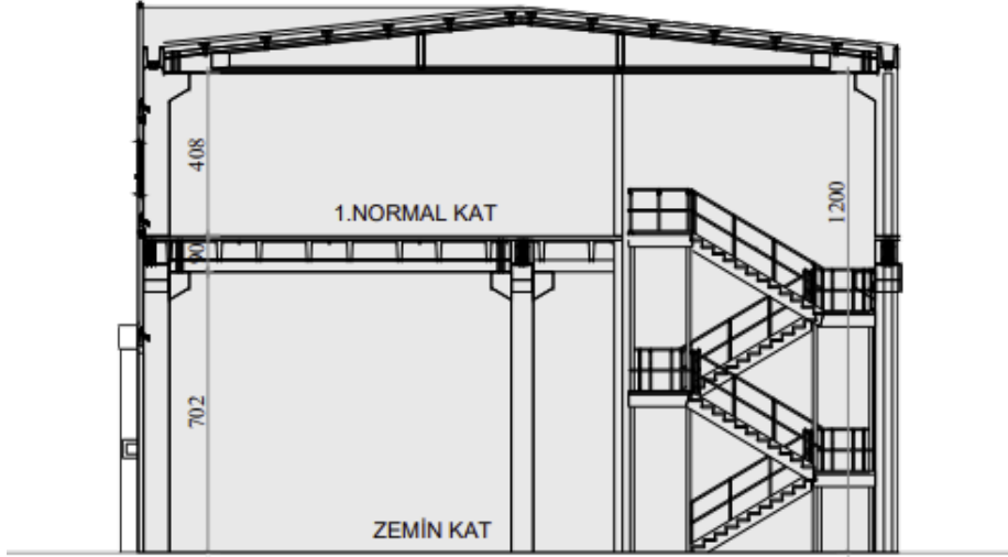
ŞEMATİK KESİT
