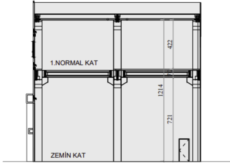
ŞEMATİK KESİT
