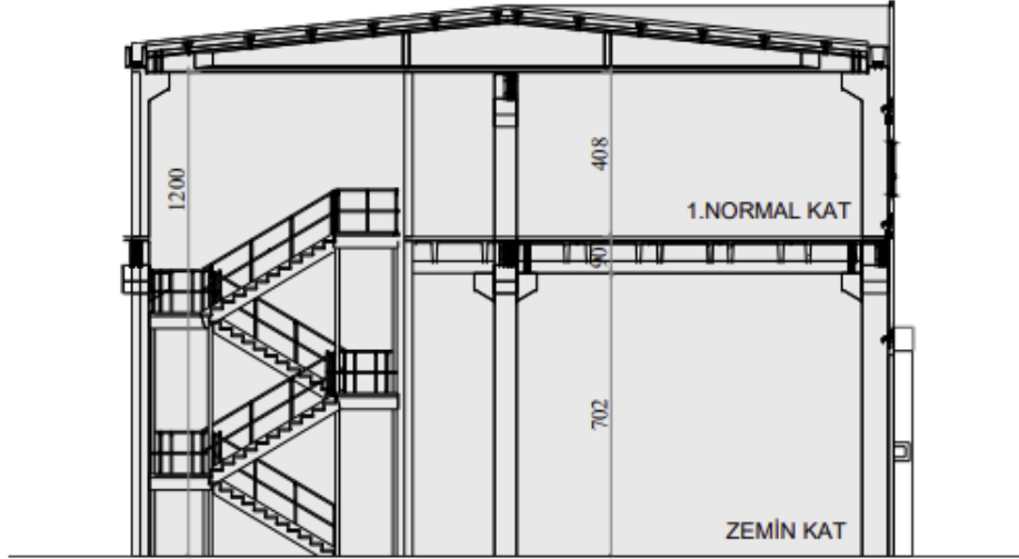
ŞEMATİK KESİT
