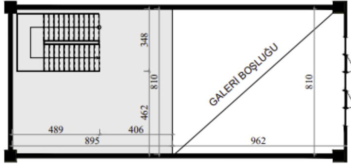
1.NORMAL KAT
