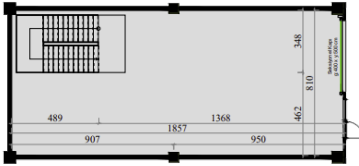
ZEMİN KAT
